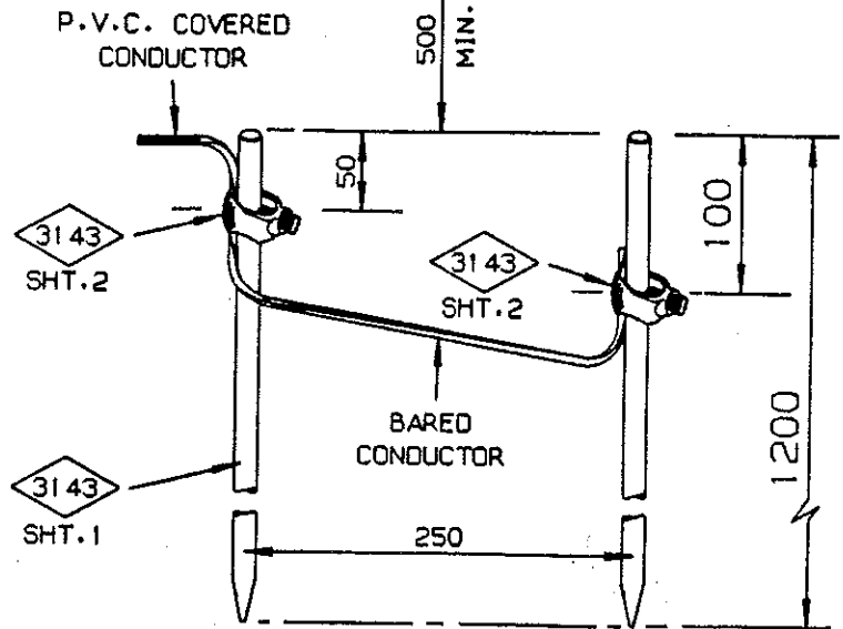
DETAIL OF EARTHING ELECTRODES. (N.T.S.)
